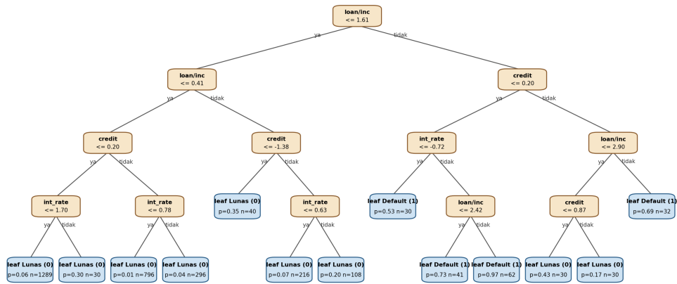
Percabangan CART dari scratch (max_depth=4), split memakai Gini gain berbobot kelas
